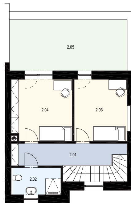
Pôdorys poschodia
