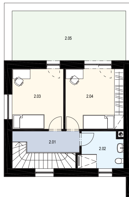
Pôdorys poschodia
